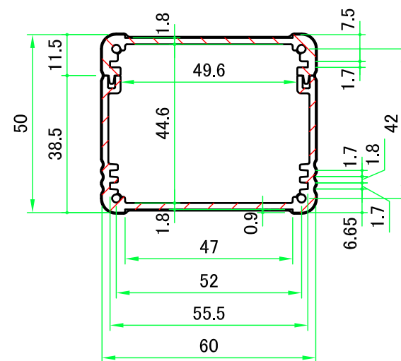
A-A ( 1 : 1.5 )
